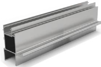
Üst Kasa Profili Ürün Kodu: 2069 Ağırlık kg/m: 2,054 (50 x 141 x 1,5mm)
