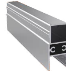
22mm Dikme ve Alt Profili Ürün Kodu: 3064 Ağırlık kg/m: 1,030 (57,5 x 27 x 1,7mm)
