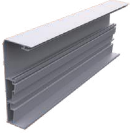
Kış Bahçesi Arka Askı Ürün Kodu: 2532 Ağırlık kg/m: 2,651 (191 x 69 x 1,8mm)
