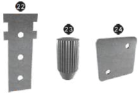
Kasnak Kayış Sıkıştırma T Sac Ürün Kodu: GYT-22 Set İçeriği: 4 Adet Kayış Bağlantı Pimi Ürün Kodu: GYT-23 Set İçeriği: 2 Adet Kayış Alt Sıkıştırma Ürün Kodu: GYT-24 Set İçeriği: 4 Adet
